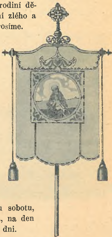
Obr. 37. Korouhev.
