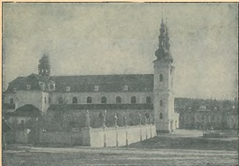
Obr. 38. Velehrad (Velehrad).
