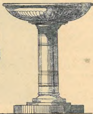
Obr. 10. a 11. Kropenky.
