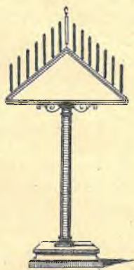
Obr. 34. Trojhranný svícen.
