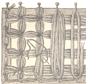
Obraz čís. 54. 2. Půda mřížovaná. Podvojnĕ zaklesnutí.
