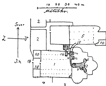
Pádorys chrámu a jeskyně Narození Páně.
