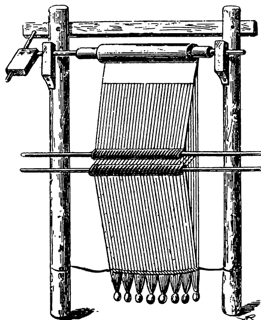
Obr. 340. Tkací stroj (řecký).
