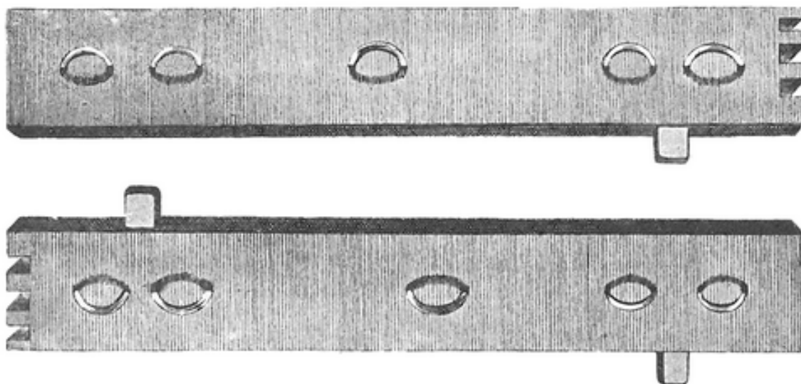
Obr. 183. Fošny stěn svatostánku.
