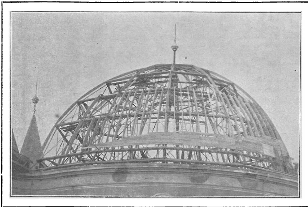
Dohotovená montáž bání kostela.
