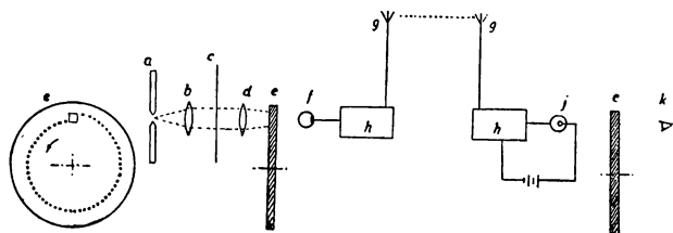
Obr. 2. Televisní systém s Nipkovovým kotoučem.
