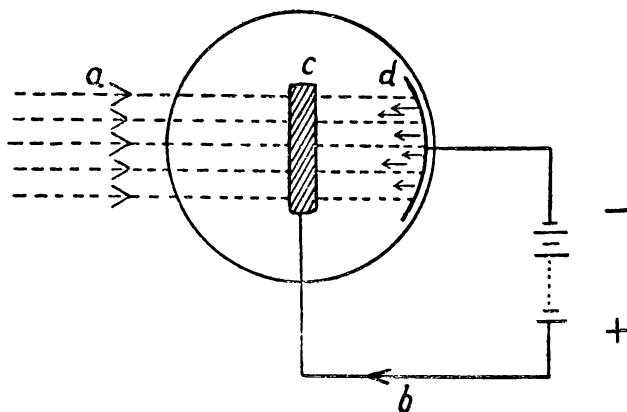
Obr. 1. a) směr světla, b) směr proudu, c) anoda, d) vystupující elektrony.
