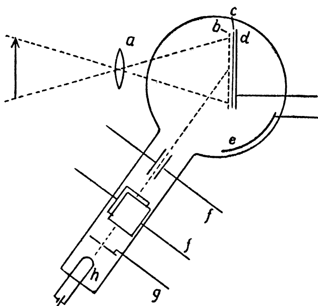
Obr. 4. Zvorykinův ikonoskop.
