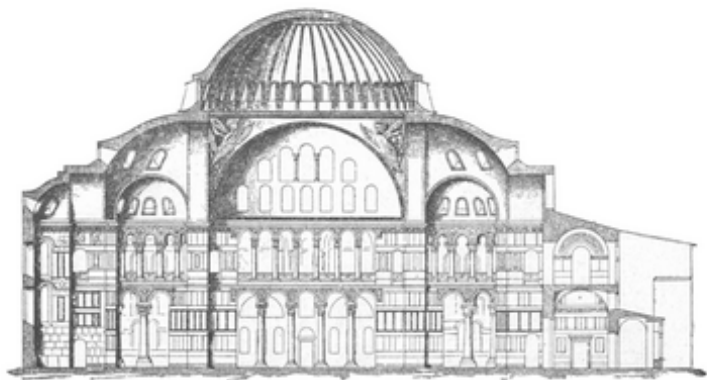
Obr. 3. Chrám Boží Moudrosti v Cařihradě; řez podélný
