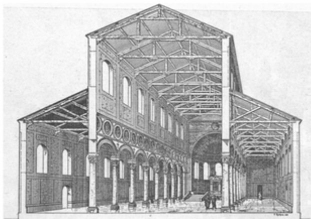
Obr. 10. Basilika sv. Apollináře v Classe u Ravenny; řez příčný.
