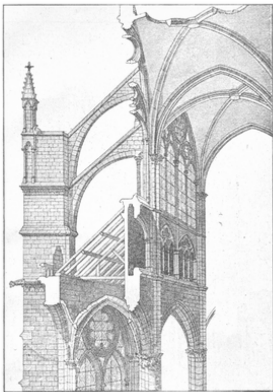
Obr. 32. Opěrný systém gotický dómu amienského.
