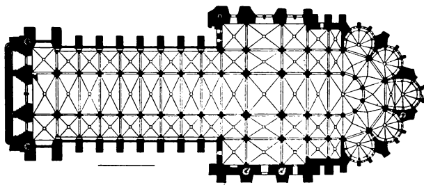
Obr. 33. Půdorys dómu remešského.
