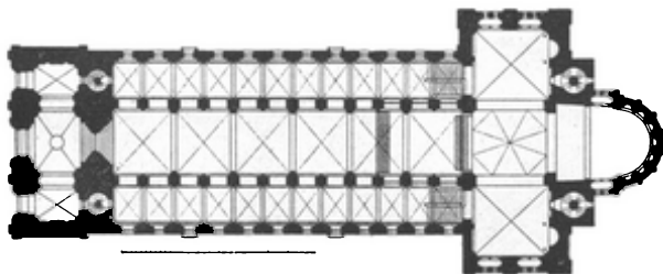
Obr. 20. Románský dóm ve Špýru; půdorys.
