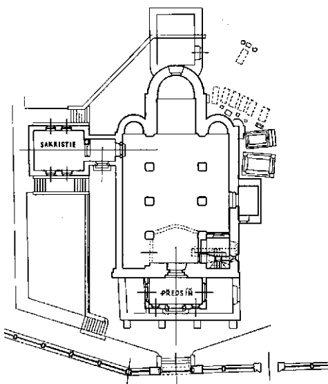
Prosek. Kostel sv. Václava. Půdorys s vyznačením starého i nového stavu.
