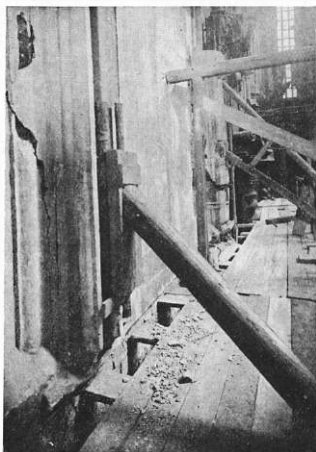
Poškozené přípory severní stěny.
