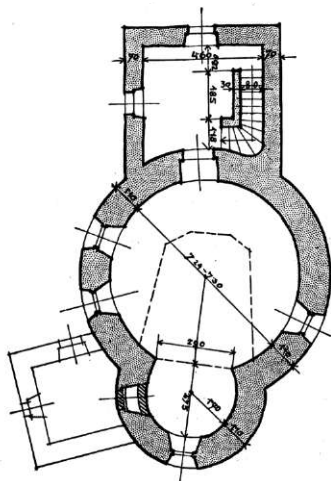
Česká Třebová: Rotunda sv. Kateřiny. Celkový pohled a půdorys.
