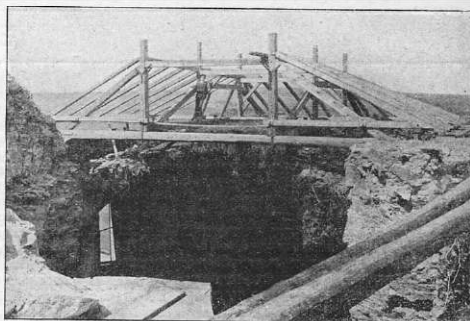
Mariánská Týnice. Pohled do vnitřní kopule po druhém zřícení roku 1920. Počátek montáže provisorní střechy.
