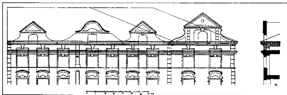
Návrh stavitele Jana Bělského na odstranění štítu domu čp. 603-I, na Staroměstském nám. (Zrnité vyznačeno, jest přestavba, provedená r. 1859.)
