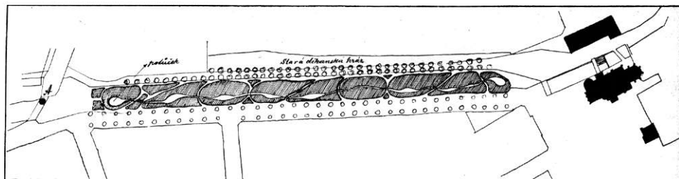
Obr. 6. Schema návrhu na úpravu vysušeného náhonu. S bodu A provedena fotografie pro obr. 5.
