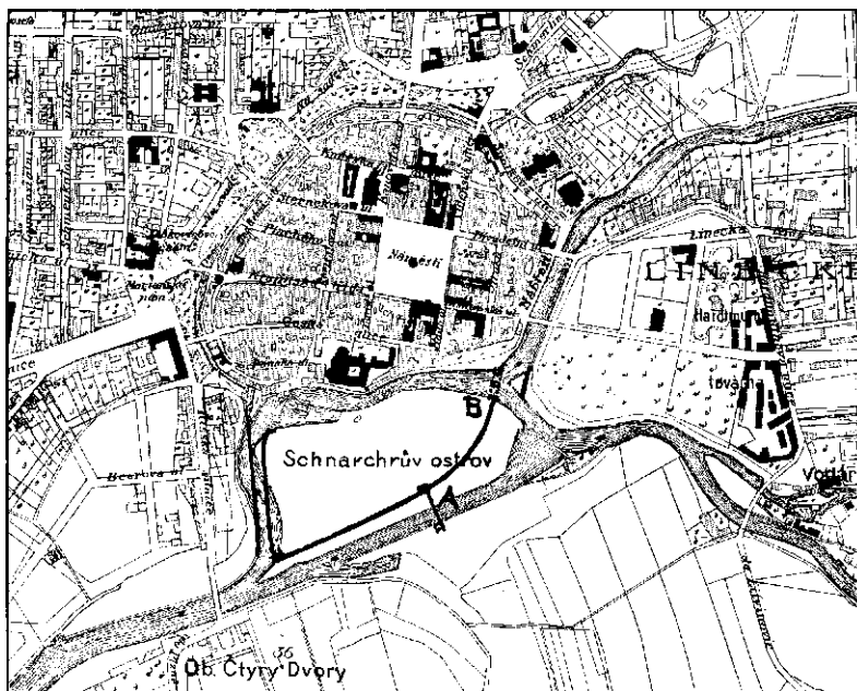
Obr. 24. Návrh Klubu umožňuje zachování hlavního ramene Vltavy uzavřením braty v místě B a užitím jediného pohyblivého jezu společného místo dvou jezů zvláštních na Malši a na Vltavě.
