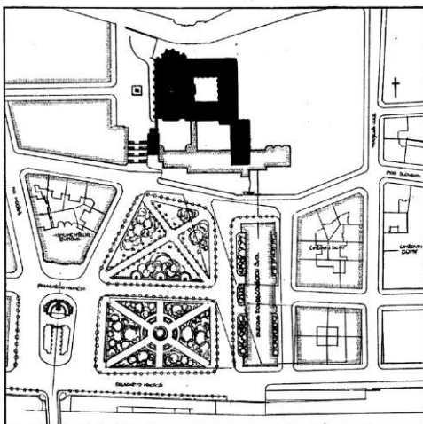
Obr. 6. Al. Dryák: Návrh na úpravu prostranství před Emauzy. (1912.) Varianta I. Púdorys.
