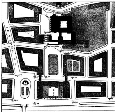
Obr. 2. VI. Hofman: Návrh na úpravu prostranství před Emauzy. (1913.) Půdorys.
