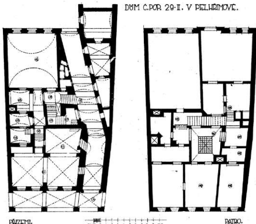
Obr. 77. Půdorys přízemí a I. patra bývalého hotelu Rosolova v Pelhřimově. Vyměřeno r. 1913.
