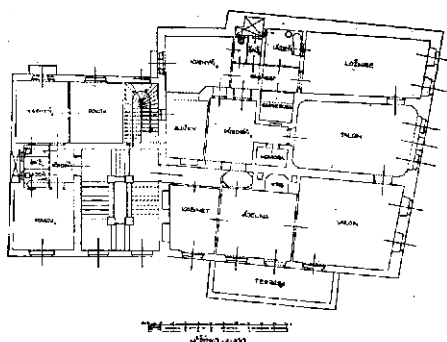
Obr. 44. Půdorys domu Demartinova podle návrhu na úpravu. První patro.
