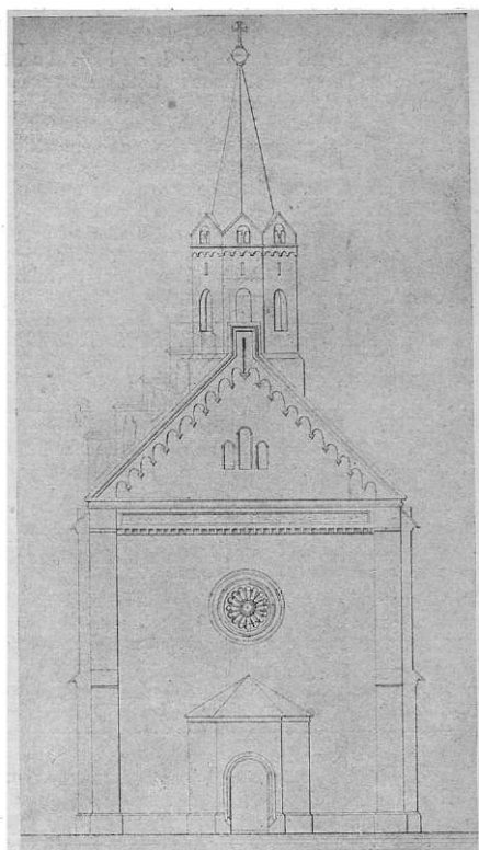
Obr. 72. P. L. Holeček: Návrh na přístavbu rotundy v Přední Kopanině. (Nárys průčelí.)
