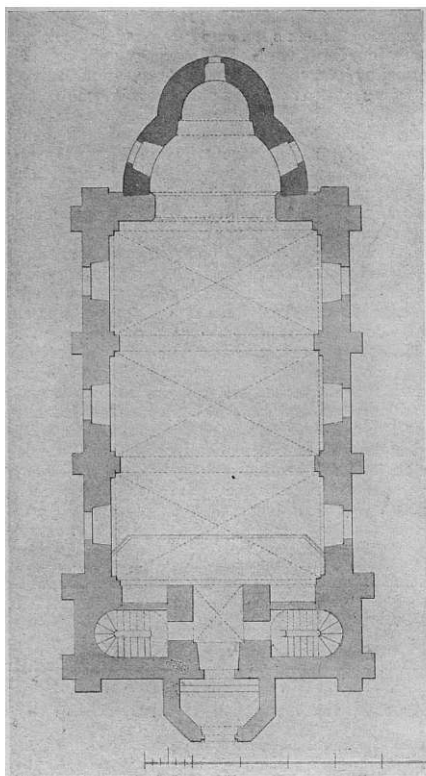
Obr. 71. P. L. Holeček: Návrh na přístavbu rotundy v Přední Kopanině. (Půdorys.)
