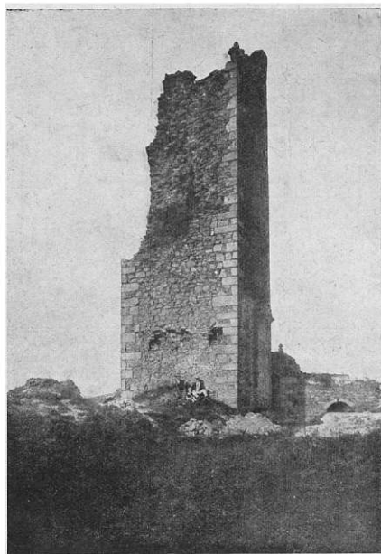
Obr. 92.-93. Zřícenina hradu Orlika u Humpolce. Stav před konservací v létě 1913.
