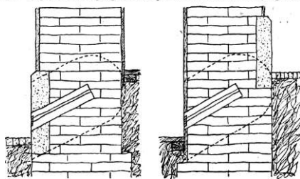
Obr. 7. Vysušení zdi podle systému Knapenova.
