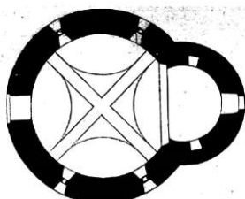
Obr. 70. Půdorys rotundy v Přední Kopanině s barokním oknem. Vynesl P. L. Holeček.
