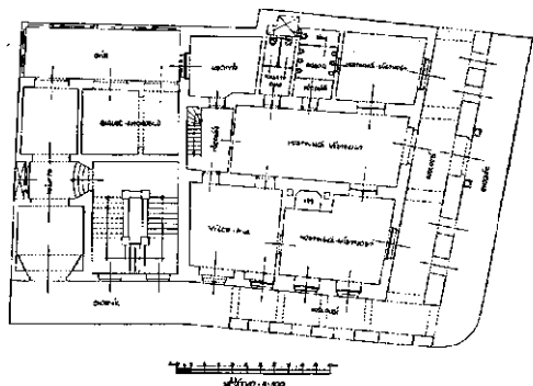
Obr. 43. Půdorys domu Demartinova podle návrhu na úpravu. Přizemí.
