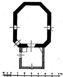
Obr. 102. Půdorys sakristie kaple P. Marie „Na šancích“.
