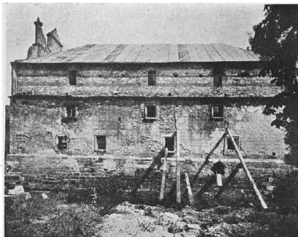
Obr. 89. Mlýn v Pátku. První období adaptace: budova měla být ve zdivu jenom zvýšena a původní zdi se šitly ponechány. (Návrh stav. V. Hrona).
