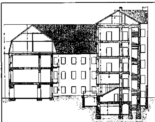
Obr. 68. Řez starým, zachovaným traktem uličním a navrženou novostavbou ve dvoře.
