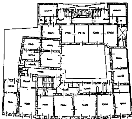
Obr. 67. Půdorys I. patra. Navržená adaptace starého traktu a rozdělení místností v navržené novostavbě ve dvoře.
