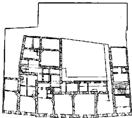
Obr. 66. Půdorys I. patra. Starý dům s původním rozdělením místností a komunikací po pavlači.
