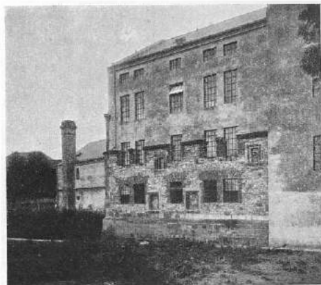
Obr. 92. Mlýn v Pátku po provedené přestavbě. Pohled na novou imitovanou návodní zeď se zasazenými starými ostěními.
