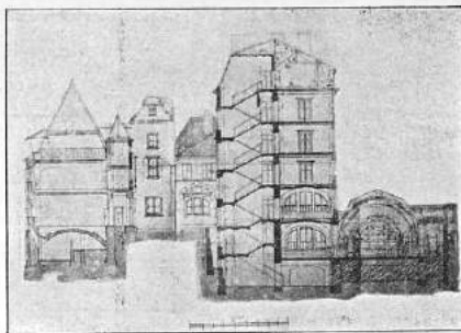
166. ŘEZ ADAPTOVANÝM DOMEM U VEJVODŮ S VESTAVĚNÝM NOVÝM DOMEM VE DVŮŘE.
