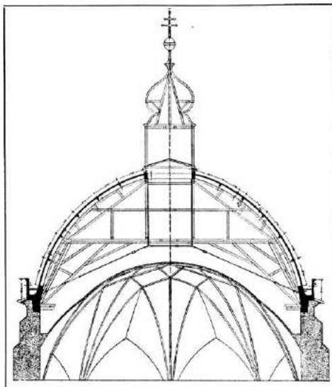
130. NÁVRH INŽENÝRŮ DOC. K. HERZÁNA A DRA A. LEDERERA NA REKONSTRUKCI KROVU KARLOVA V ŽELEZOBETONU: ŘEZ STARÝM KROVEM, NA NĚMŽ MÁ BÝT VYBETONOVÁN NOVÝ ŽELEZOBETONOVÝ KROV.
