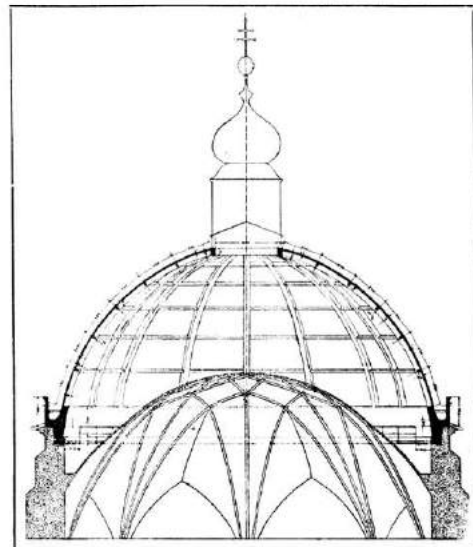
131. NÁVRH INŽENÝRŮ DOC. K. HERZÁNA A DRA A. LEDERERA NA REKONSTRUKCI KROVU KARLOVA V ŽELEZOBETONU: ŘEZ NOVÝM ŽELEZOBETONOVÝM KROVEM PO ODSTRANĚNÍ STARÉHO VADNÉHO DŘEVĚN. KROVU.
