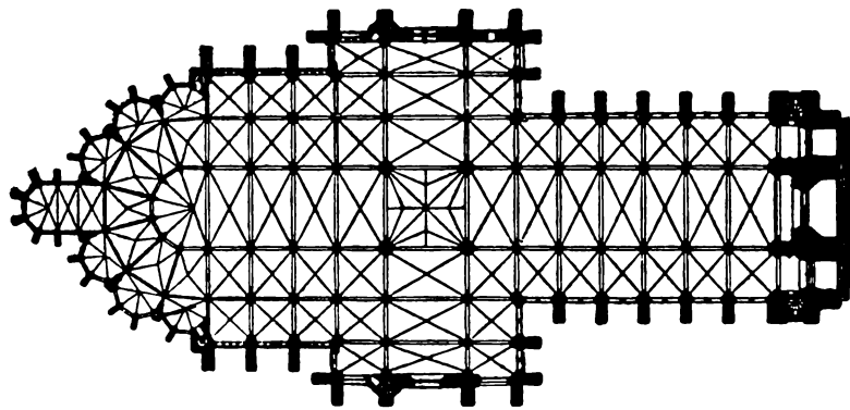
18. Opěrná soustava katedrály amienské. — 19. Púdorys katedrály amienské.
