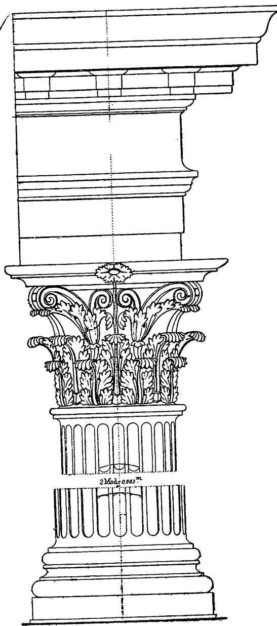
Obr. 11. Sloup korintský.
