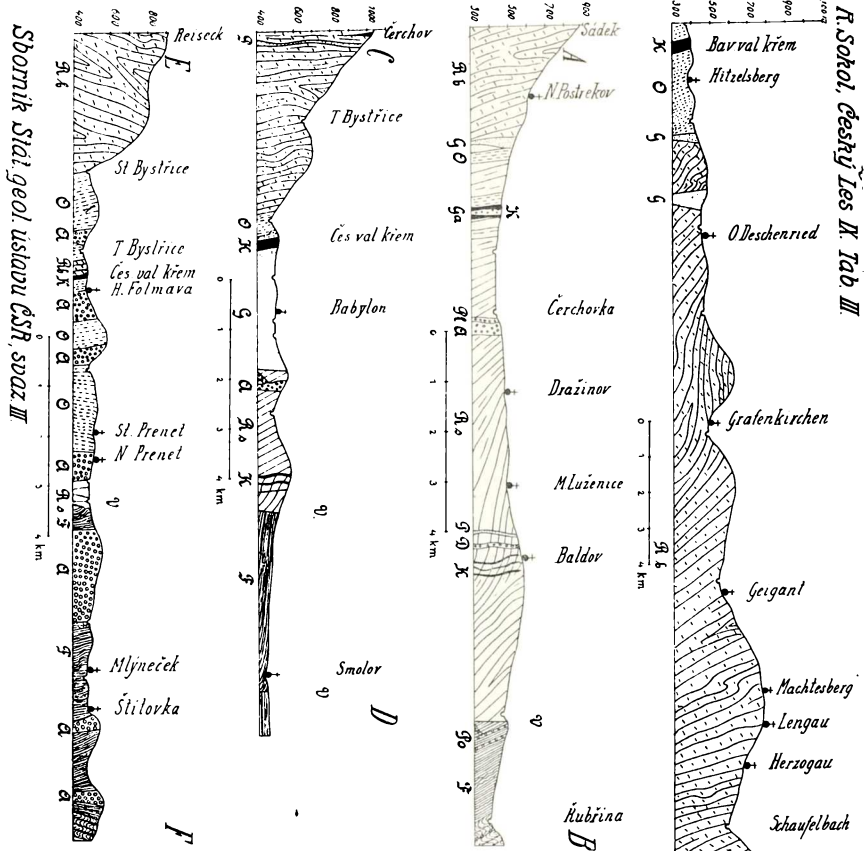
Obr. 13. Průřezy Českým Lesem. Horní veden v Bavořích od Hitzelsbergu k Čerchovu, ostatní tři českou částí Českého Lesu: AB od Nového Postřekova k Milavčím, CD od Čerchova k Smolovu, EF od Reisecku (Rejsku) v Bavořích k Štítovce. G žula, P pegmatit, Po porfyr, A amfibolit, D diorit, Pl plagioplit, Ga gabbro, K křemenný aplit, křemen (na Čerchově erlán). Rb rula biotitová, Rs rula sivorová, F fylit, O orthurla, V zlomy.
